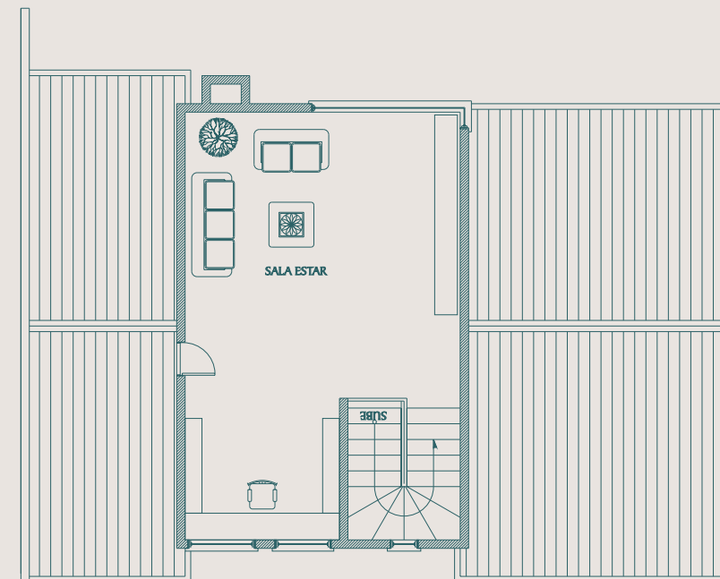
PLANTA ALTILLO
