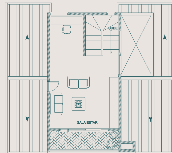
PLANTA ALTILLO
