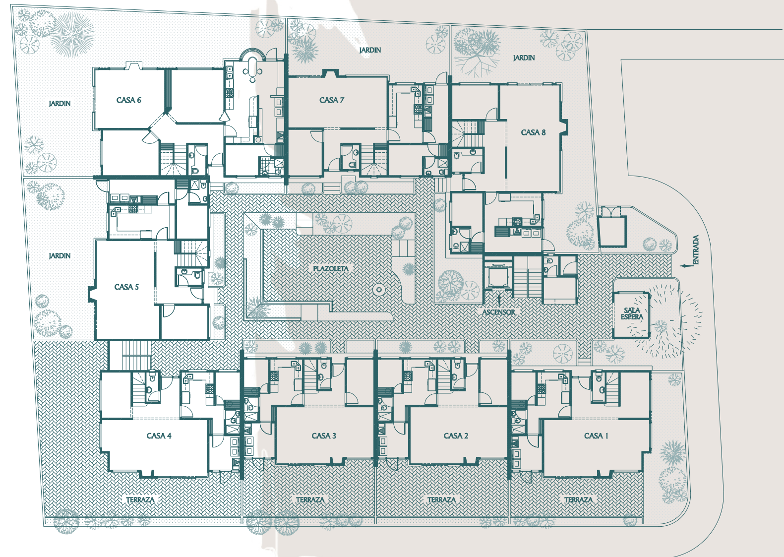
PLANTA GENERAL DEL CONJUNTO
