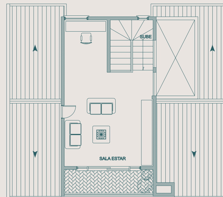
PLANTA ALTILLO
